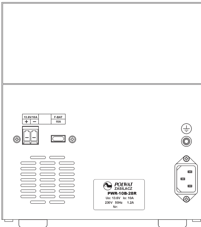
Rys.2. Panel przyłączeniowy zasilacza PWR-10B-28R
