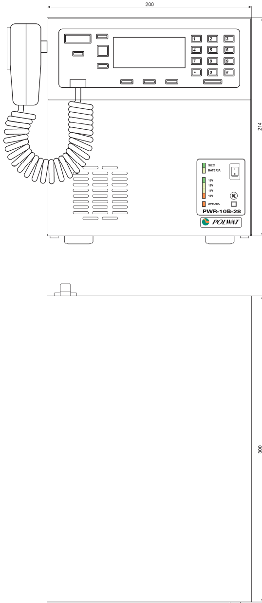
Rys.3. Wymiary gabarytowe zasilacza PWR-10B-28R
