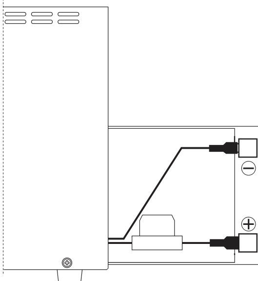
Rys.3. Wymiana akumulatora
