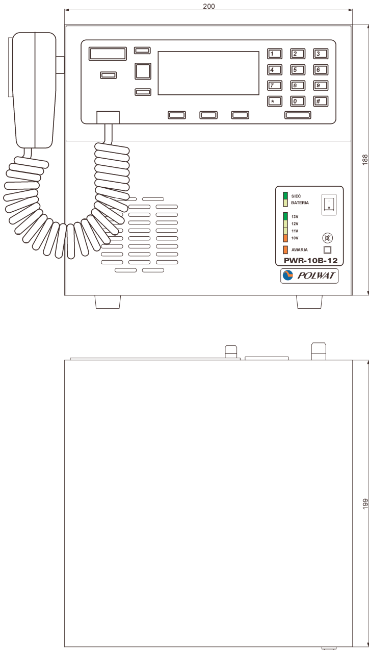
Rys.4. Wymiary gabarytowe zasilacza PWR-10B-12R
