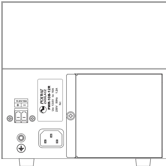
Rys.2. Panel przyłączeniowy zasilacza PWR-10B-12R
