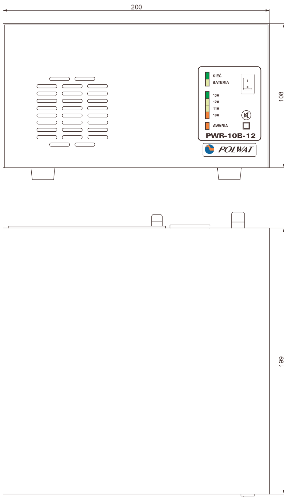
Rys.1. Wymiary gabarytowe zasilacza PWR-10B-12
