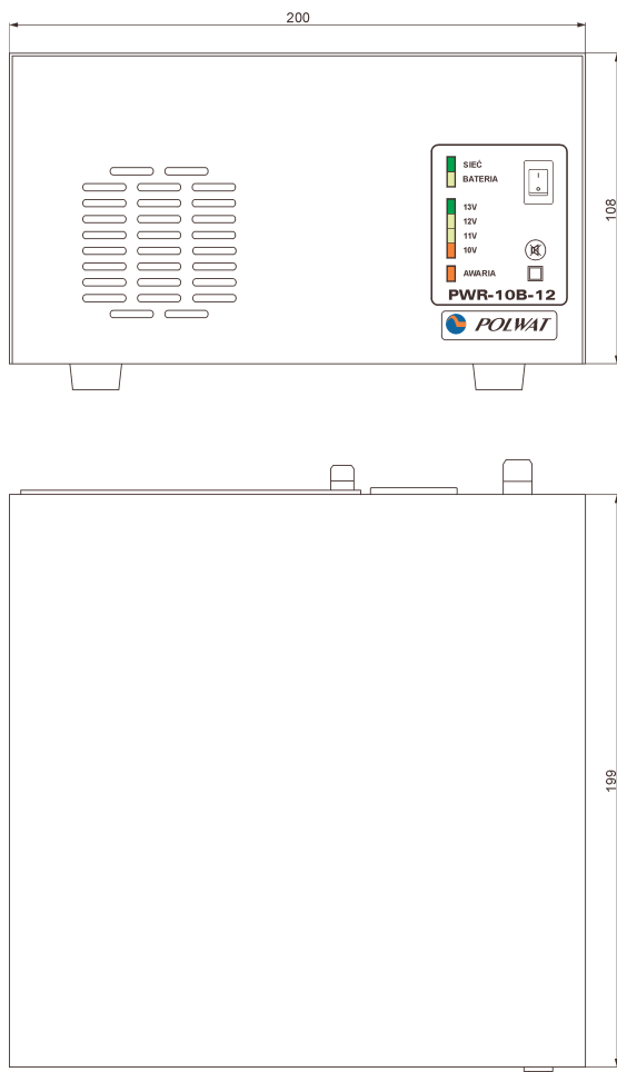
Rys.4. Wymiary gabarytowe zasilacza PWR-10B-12
