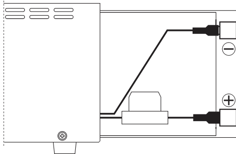
Rys.3. Wymiana akumulatora.
